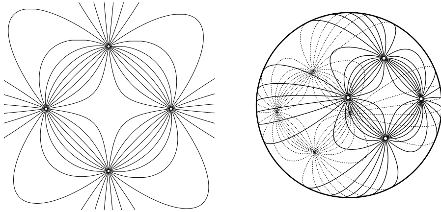
Abbildung 6: Scharen von Kegelschnitten durch vier Punkte.
