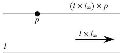
Abbildung 4: Berechnung einer Parallelen.
