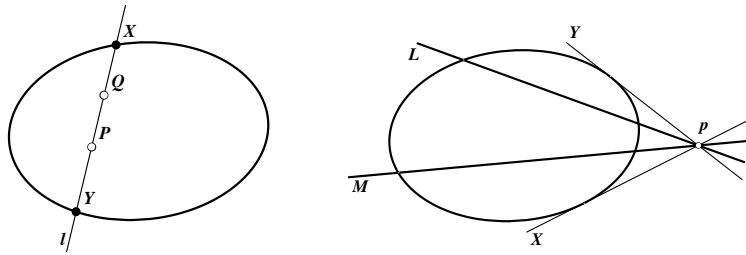
Abbildung 11: : Zur Maßbestimmung in Cayley-Klein Geometrien.
