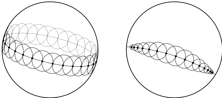
Abbildung 13: Kreise gleicher Größe in elliptischer und hyperbolischer Geometrie. Darstellung auf der Kugeloberfläche und in der Poincaré'schen Kreisscheibe.
