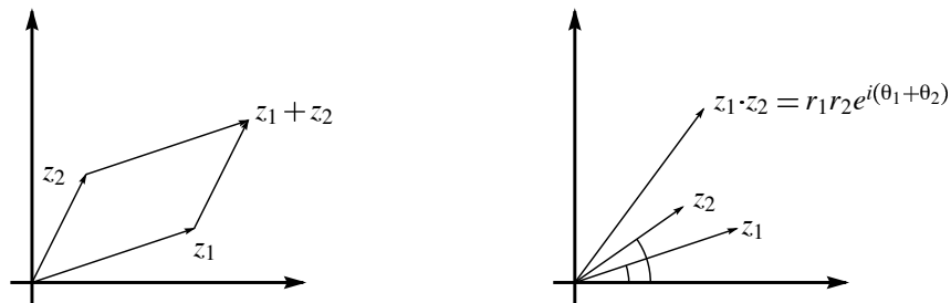
Abbildung 10: Addition und Multiplikation komplexer Zahlen.
