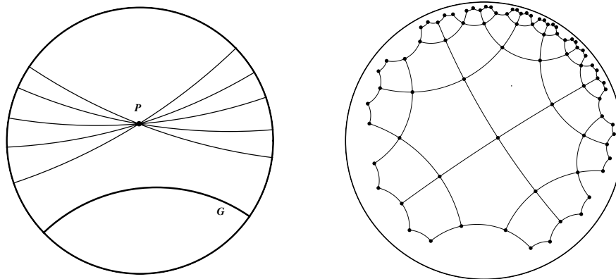
Abbildung 1: Links: Viele Parallelen einer Geraden in hyperbolischer Geometrie. Rechts: Parketierung der hyperbolischen Ebene mit "gleichgroßen" Fünfecken.
