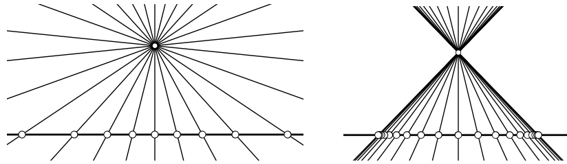
Abbildung 12: Strahlen auf äquidistante Punkte in elliptischer und hyperbolischer Längenmessung.
