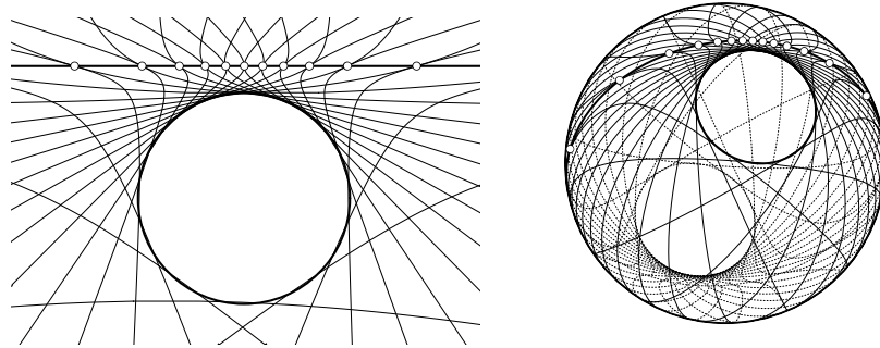
Abbildung 14: “Kreise” gleicher Größe in elliptischer Maßbestimmung auf einer Geraden, die in hyperbolischer Geometrie die hyperbolische Kreisscheibe nicht schneidet. Für Experten und Ästheten.
