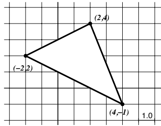
Abbildung 5: Flächenberechnung eines Dreiecks.
