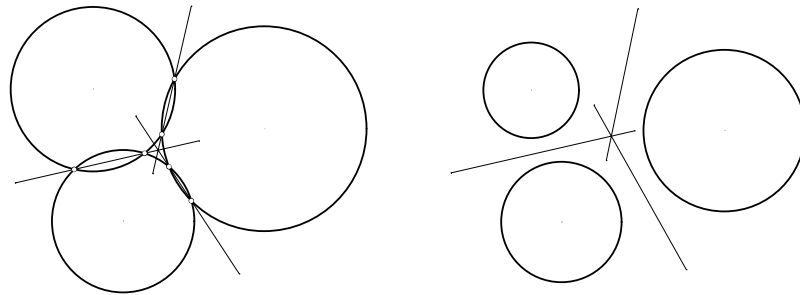
Abbildung 8: Gegeben seien drei Kreise. Für jedes Paar zieht man die Verbindungsgerade der zwei Schnittpunkte. Die drei entstehenden Geraden sind reell und schneiden sich, unabhängig ob die Schnittpunkte reell sind oder komplex.
