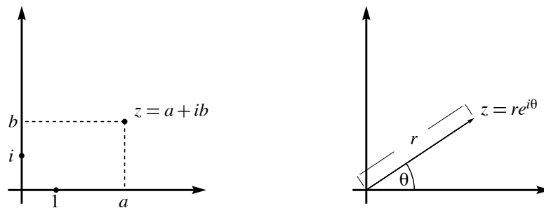
Abbildung 9: Komplexe Zahlen als Vektoren und in Polarkoordinaten.
