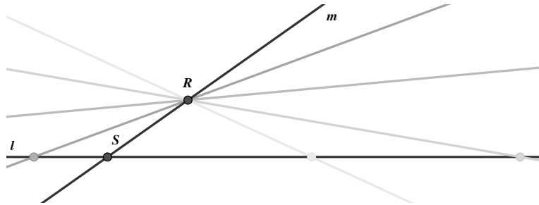
Abbildung 2: Schleifende Schnitte von Geraden verschwinden im Unendlichen und kommen von der anderen Seite zurück.
