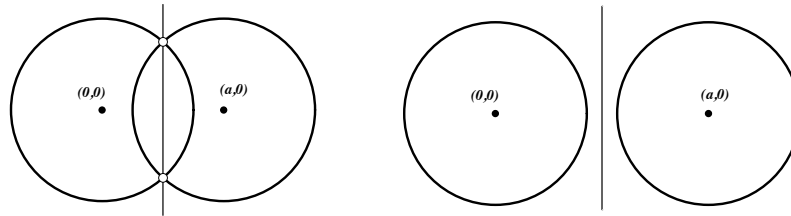
Abbildung 7: Die Verbindungsgerade der Schnittpunkte zweier Kreise ist immer reell, selbst wenn die Punkte komplex werden.
